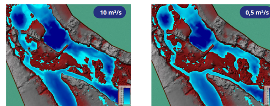
Figure 48 : Modélisation des hauteurs d'eau - scénario 4 (M.Garnault)
